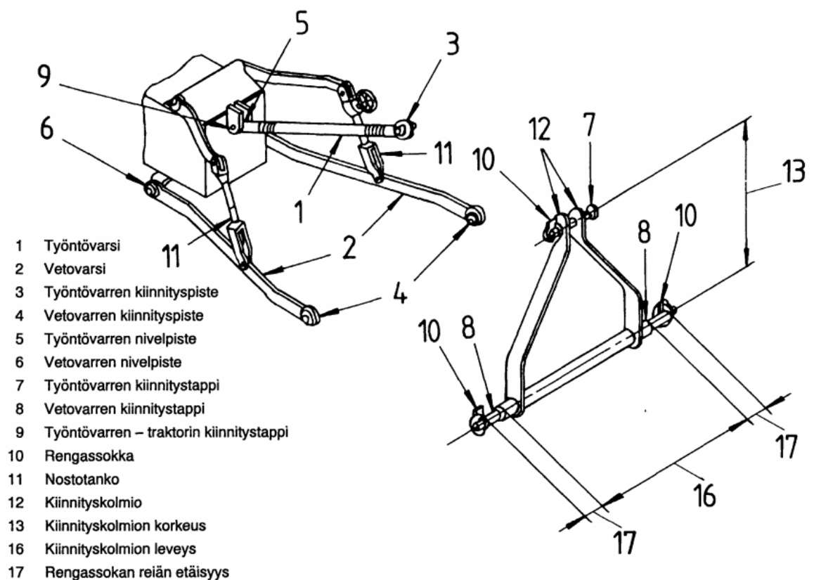
Kuva 1. Kolmipistekiinnityksen osat (SFS 1996).
