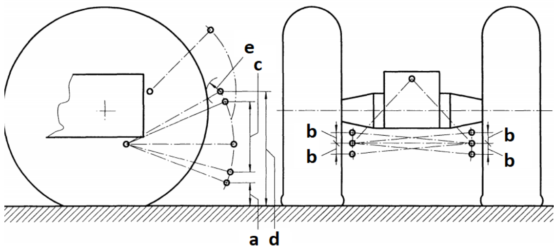
Kuva 3. Nostoalueiden ja säätövarojen määrittelyt (mukaihen SFS 1996).
